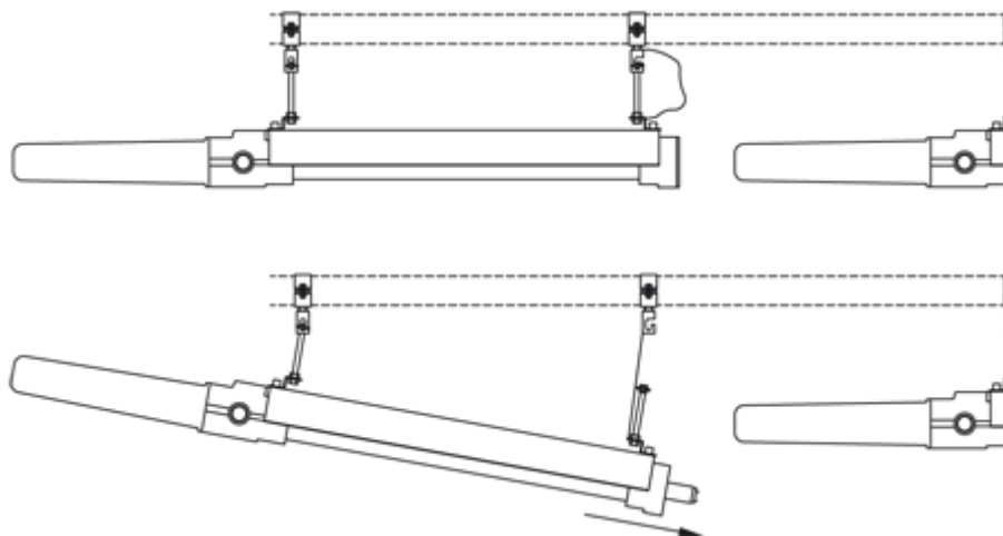
Линейная установка светильников на скобах G-0318+ G-0318/1
